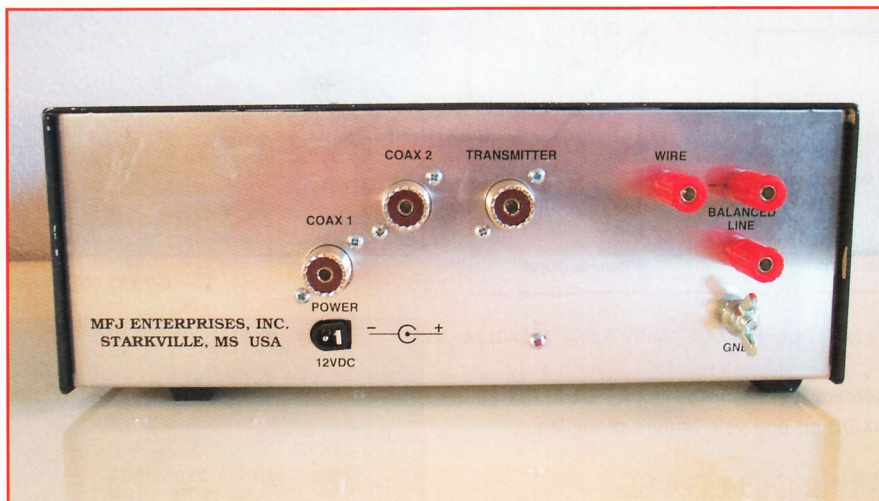
MFJ-969 achterzijde.
